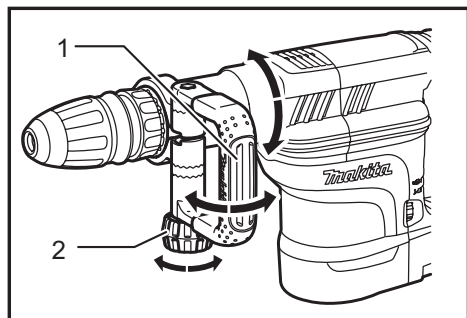
► 1. Mango lateral con forma 'D' 2. Tuerca fijadora
